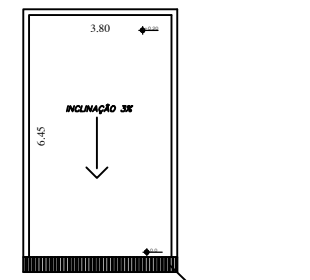
CANALETA COLETORA DETALHAMENTO GARAGEM NOVA Esc. 1:100
