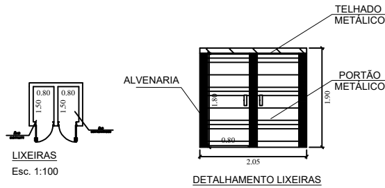
DETALHAMENTO LIXEIRAS
