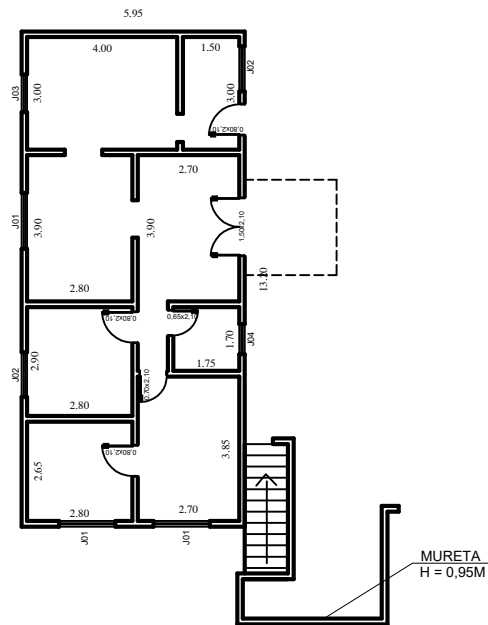
PLANTA BAIXA EXISTENTE 1º PAVIMENTO Esc. 1:100
