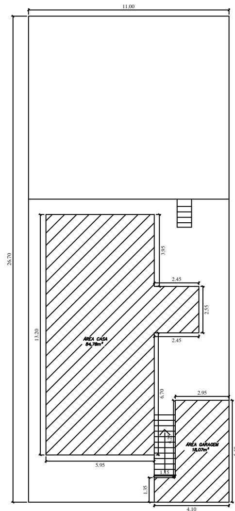
PLANTA DE LOCAÇÃO EXISTENTE Esc. 1:100
